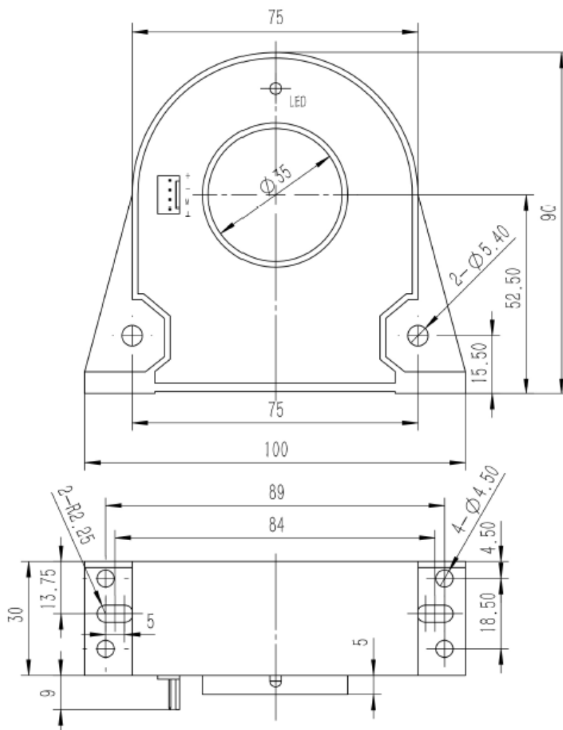
图 1 外形图
